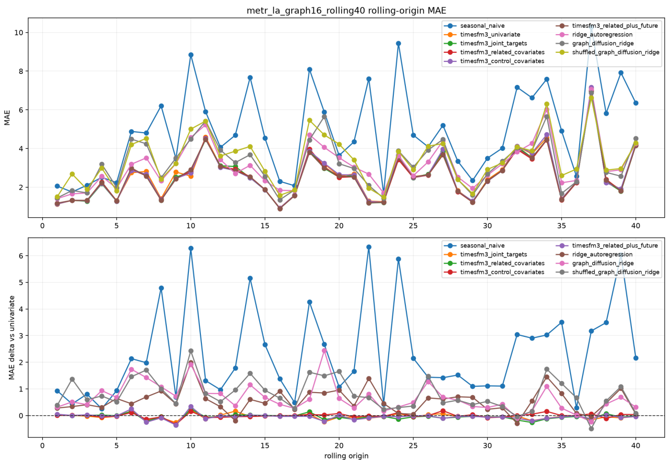
그림 3. 40개 origin별 MAE(위)와 단변량 대비 차이(아래). TimesFM 3 모드들의 차이는 0 근처에 몰려 있고, ridge 계열은 대부분 origin에서 단변량보다 위에 있다. 극단 origin(10, 24, 37)은 모든 모델에서 함께 어려웠다.
